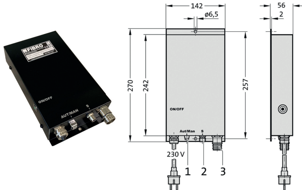
Fig. 3-2 Dimensiones unidad de control BLACK LINE
