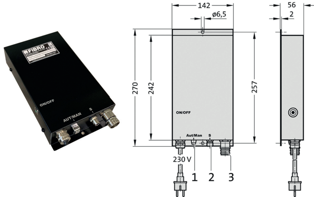
Abb. 3-2 Abmessungen Steuereinheit BLACK LINE
