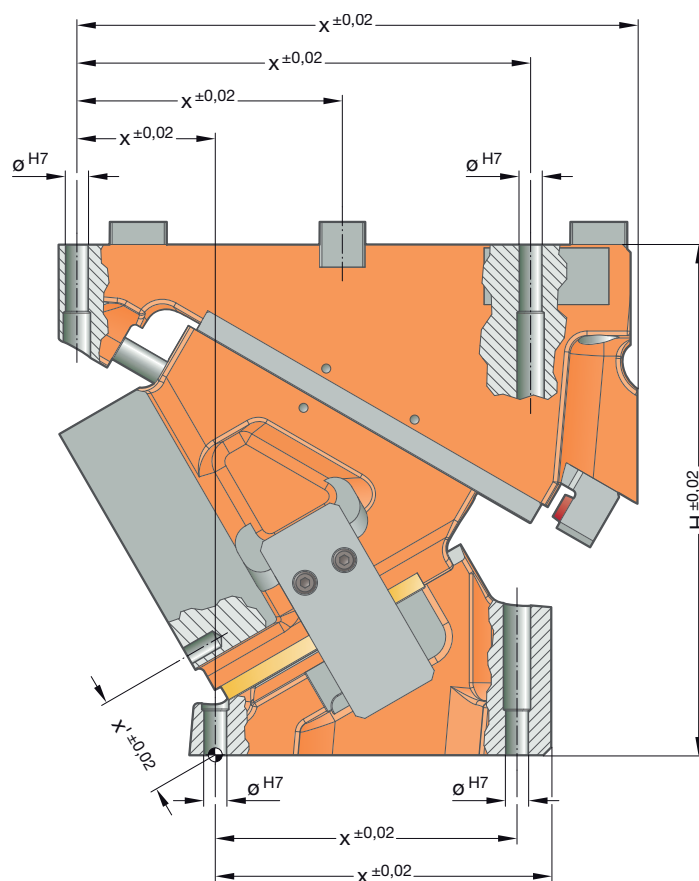
Figura 1: Tolerancias de la corredera superior con equipamiento EFP
