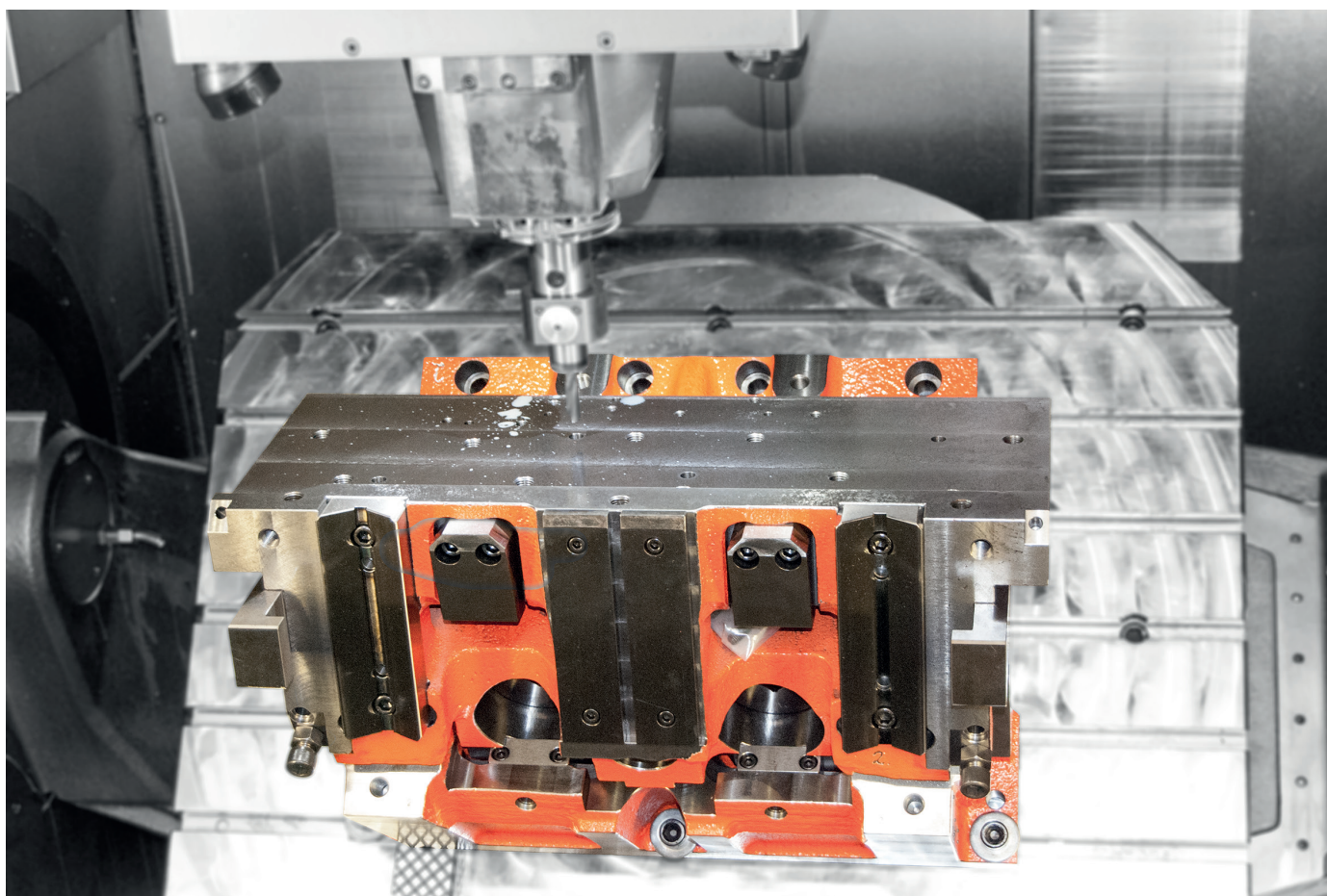
Obrázek 3: Částečné opracování klínových šoupátek podle dat zákazníka
