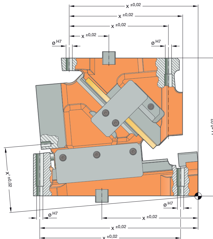
Obrázek 2: Tolerance pro zdola zavěšenou klínovou jednotku s EFP vybavením
